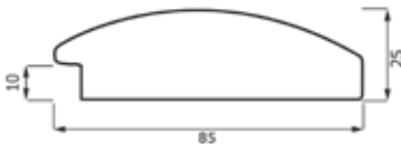
Perfil del marco | Ref. Q616
