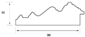
Perfil del marco | Ref. 3576
