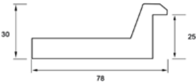
Perfil del marco | Ref. 4150
