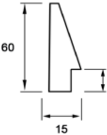
Perfil del marco | Ref. 5770 y 4016
