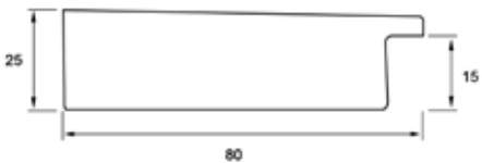
Perfil del marco | Ref. 656
