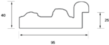
Perfil del marco I Ref. 750
