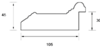
Perfil del marco | Ref. 832
