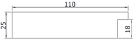
Perfil del marco I Ref. 687
