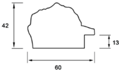
Perfil del marco | Ref. 838
