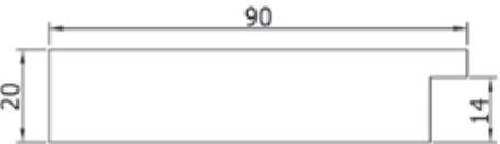
Perfil del marco I Ref. 689
