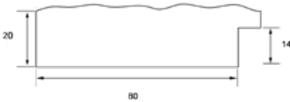
Perfil del marco I Ref. 605
