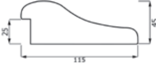
Perfil del marco | Ref. Q818
